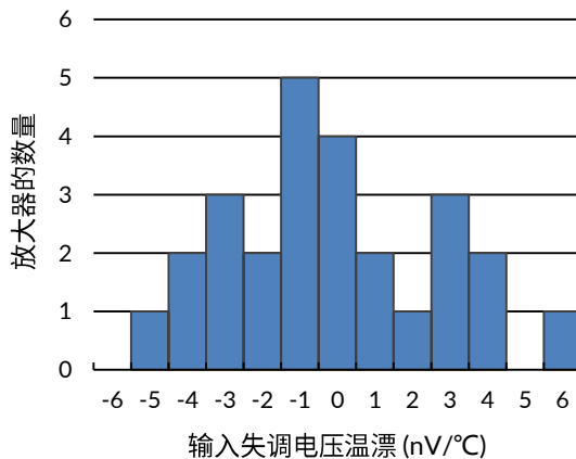
图 2. 失调电压温漂分布
