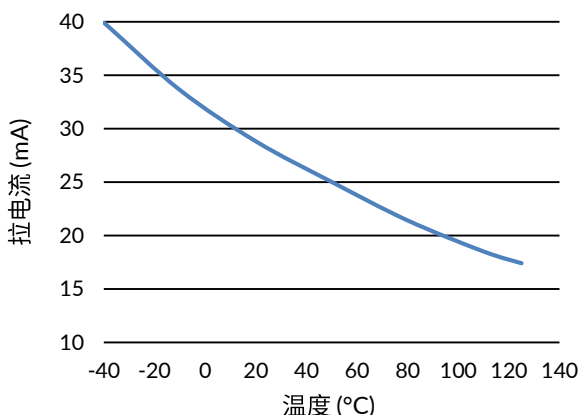
图 10. 拉电流与温度的关系
