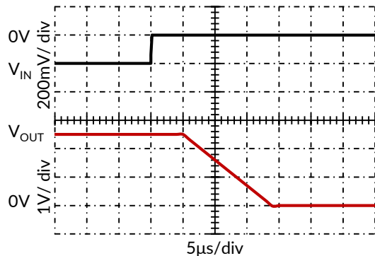
图 13. 正向过载恢复, V_S = \pm 2.5\text{V} , G = -100
